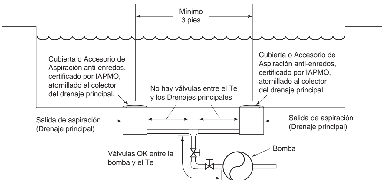
Figura 3 – Configuración recomendada de la aspiración de la bomba.
