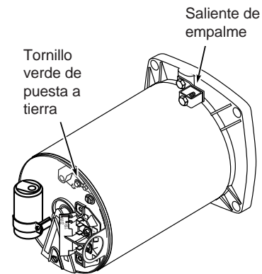
Figura 4 – Ubicaciones típicas del tornillo de puesta a tierra y de la saliente de empalme.
